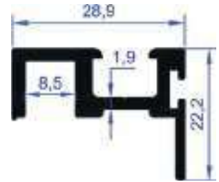
73520 Dar Yan Kulp
