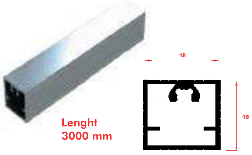
UNS-81631 30mm Ara Birleştirme UNS-81631 30mm Joining Strip
